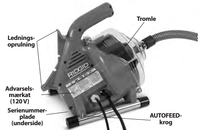
Figur 2 – PowerClear-afløbsrenssemaskine
