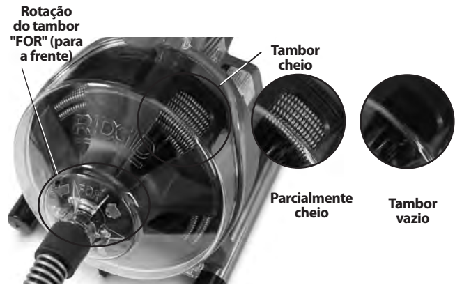
Figura 10 – Monitorizar o cabo no tambor
