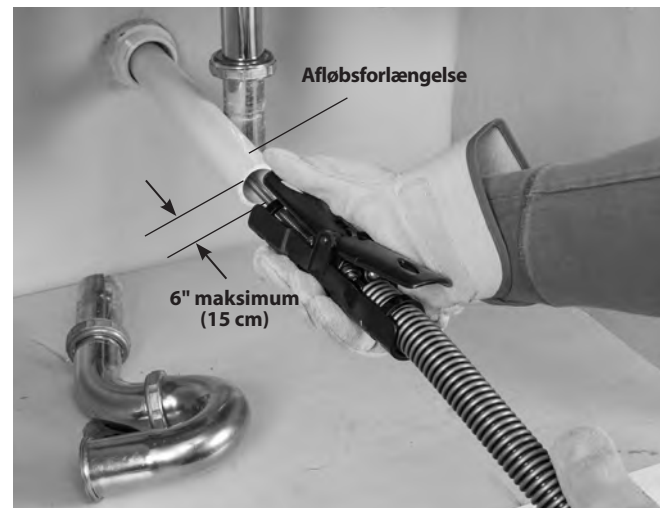
Figur 7 – Eksempel på forlængelse af afløbet til inden for en afstand af 6" (15 cm) fra AUTOFEED-enheden.
