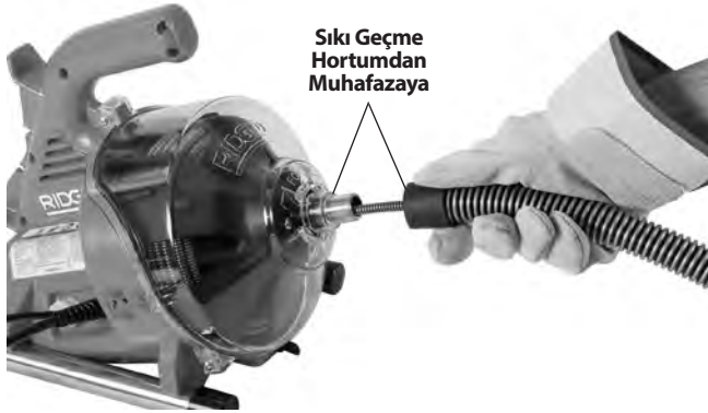
Şekil 4 – Kablo ucu kapağını Kılavuz Hortumun İçine Besleme
