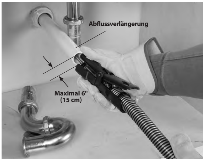
Abbildung 7 – Beispiel für eine Verlängerung des Ablaufs auf weniger als 6" (15 cm) von der AUTOFEED-Einheit
