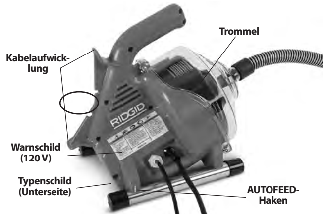
Abbildung 2 – PowerClear Abflussreinigungsmaschine
