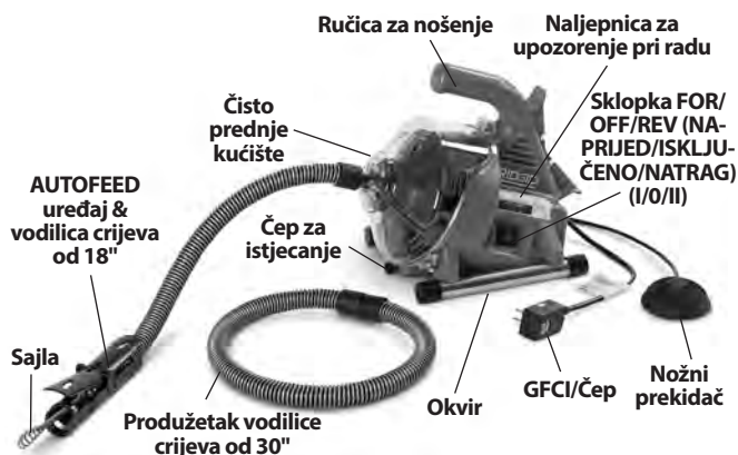
Slika 1 - PowerClear Uređaj za čišćenje odvoda
