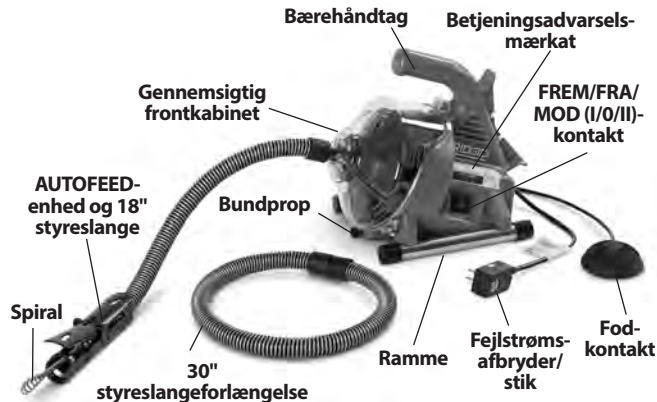
Figur 1 – PowerClear-afløbsrenssemaskine
