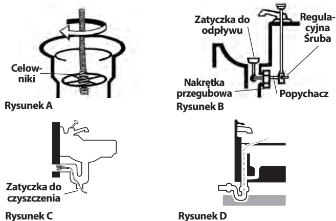
Rysunek 6 - Dostęp do odpływu
